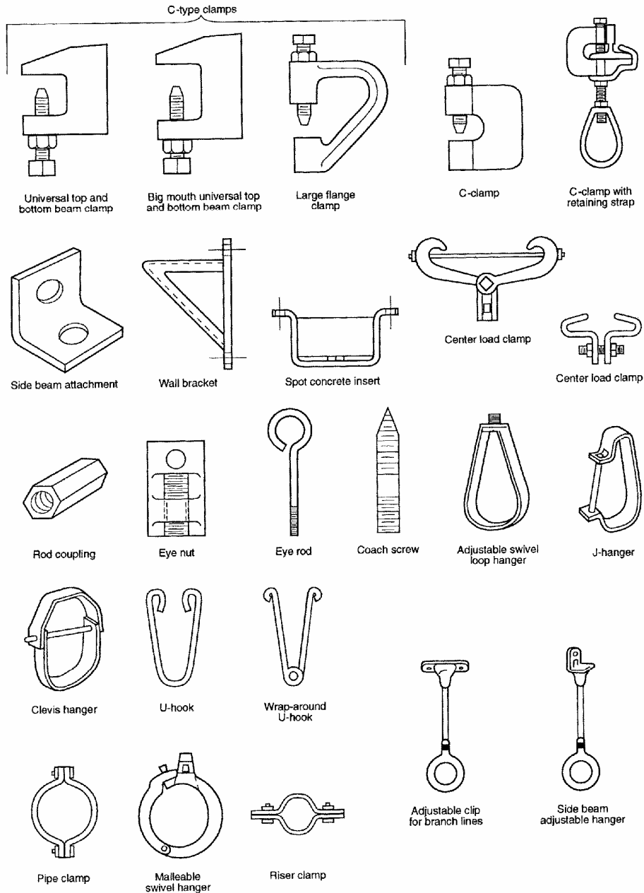
Gambar 7.9.8. : Gantungan pipa
