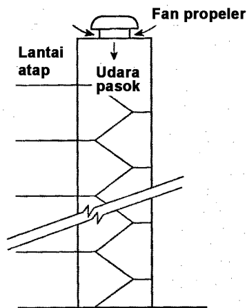
Gambar 5.3.4.1.1 : Presurisasi sumur tangga oleh fan propeler yang dipasang di atap.
