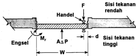
Gambar A.5.2.2 Gaya-gaya pada pintu dalam suatu pengendalian asap.
