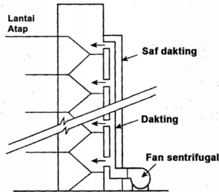
Gambar 5.3.5.2.1(a) : Presurisasi sumur tangga dengan injeksi jamak dengan fan yang ditempatkan pada lantai bawah.
