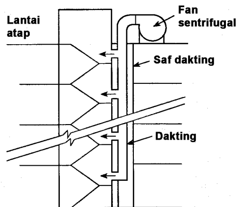
Gambar 5.3.5.2.1.(b) : Presurisasi sumur tangga dengan injeksi jamak dengan fan yang dipasang di atap.
