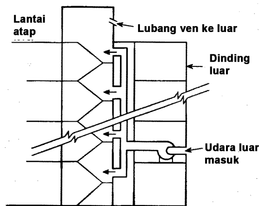
Gambar 5.3.2.2.2 : Presurisasi sumur tangga dengan ven ke luar
