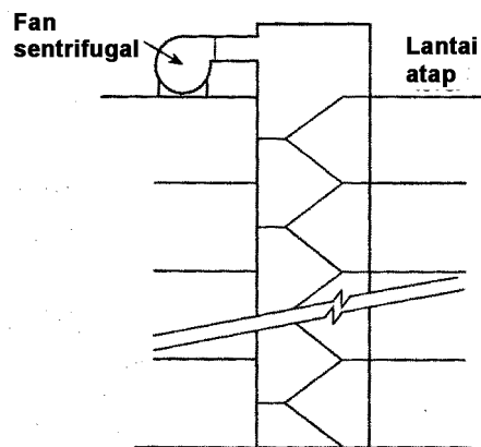
Gambar 5.3.5.1.1. : Presurisasi sumur tangga oleh injeksi di atas.
